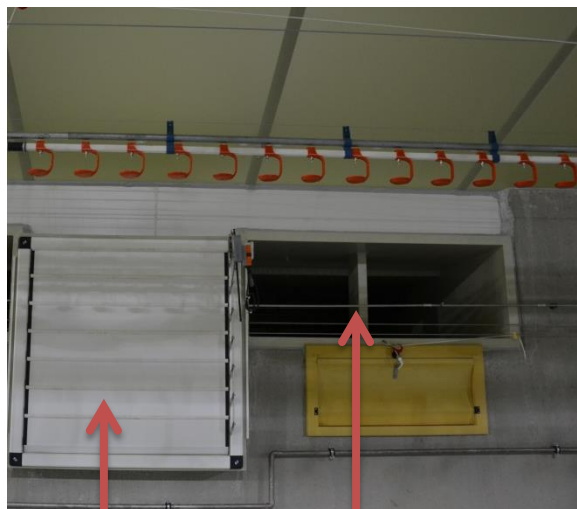
Louvreklep t.b.v. luchtinlaat
